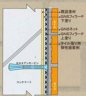
④仕上用タイル張り
